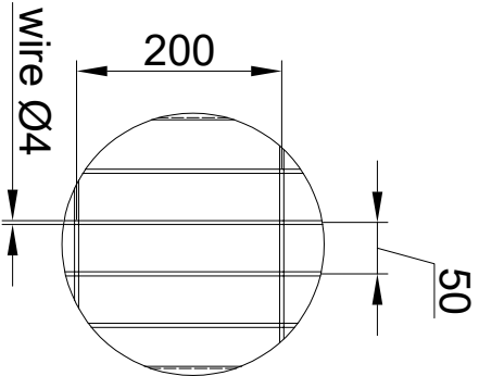
DETAIL-A (SCALE 1:1)
