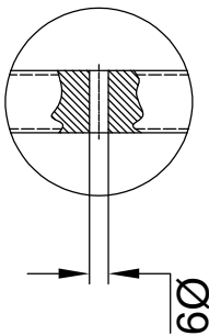
DETAIL-B (SCALE 2:1)
