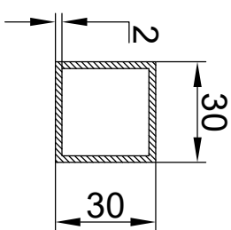
SECTION A-A (SCALE 4:1)
