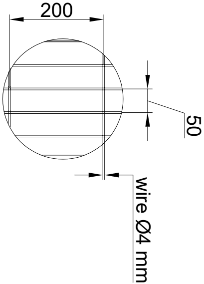
DETAIL-A (SCALE 1:1)
